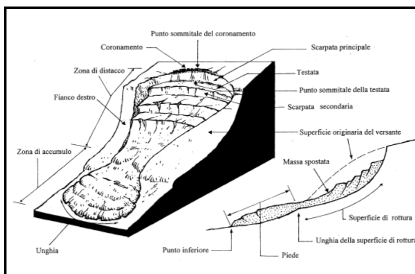
Schema della nomenclatura degli elementi di una frana (APAT – Progetto IFFI)
